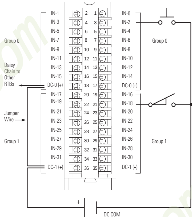
1756-IV32, 1756-IV32K
