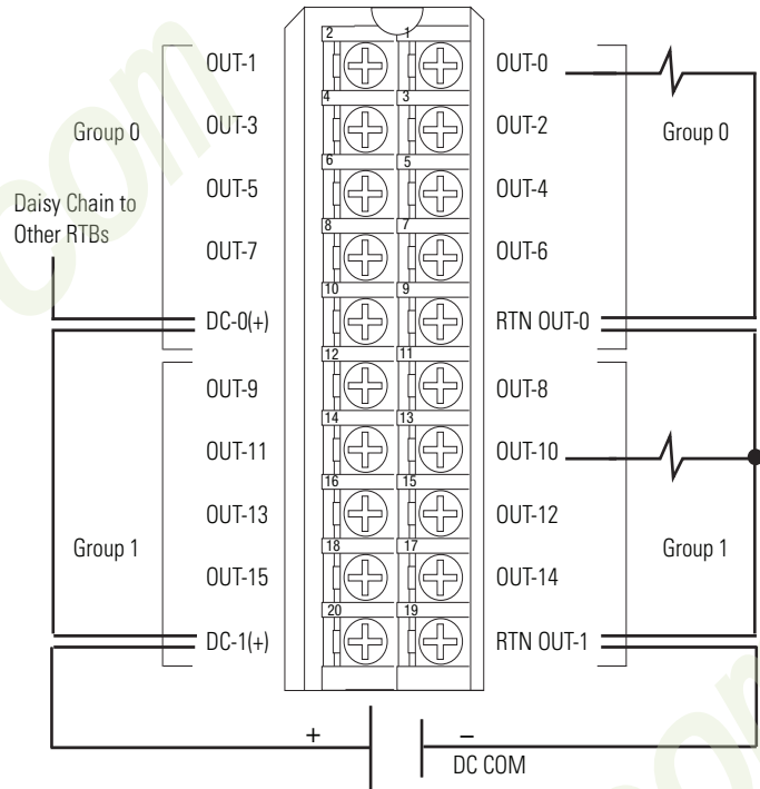
1756-OB16E, 1756-OB16EK
