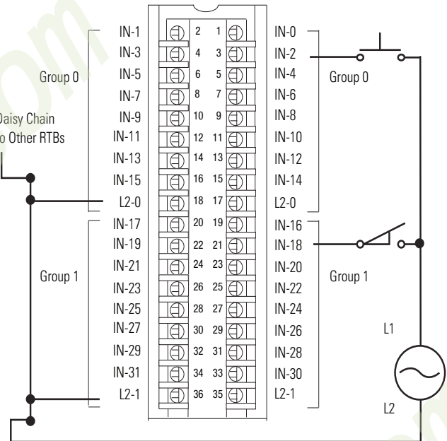
1756-IA32, 1756-IA32K
